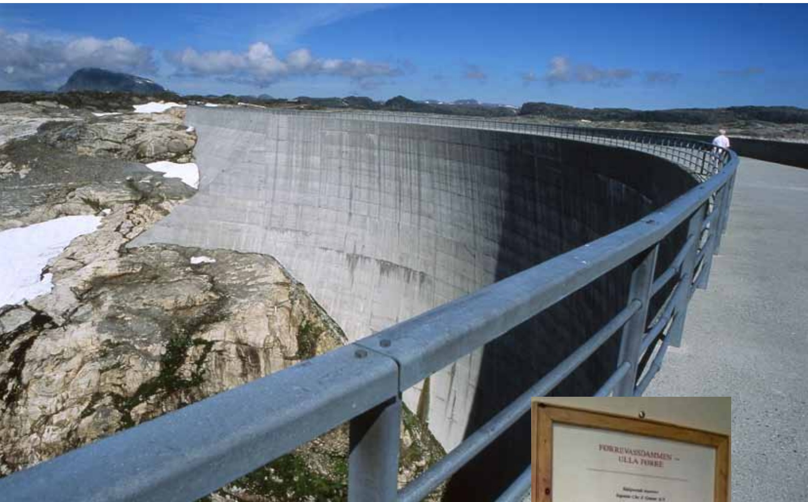
Førrrevassdammen, den største betongdammen i Norden. Foto Rune Roalkvam 1997. Til høgre "Betongtavlen", pris gitt for dette byggverket.
