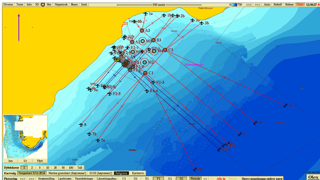
Rammer og flåter med fortøyningslinjer
